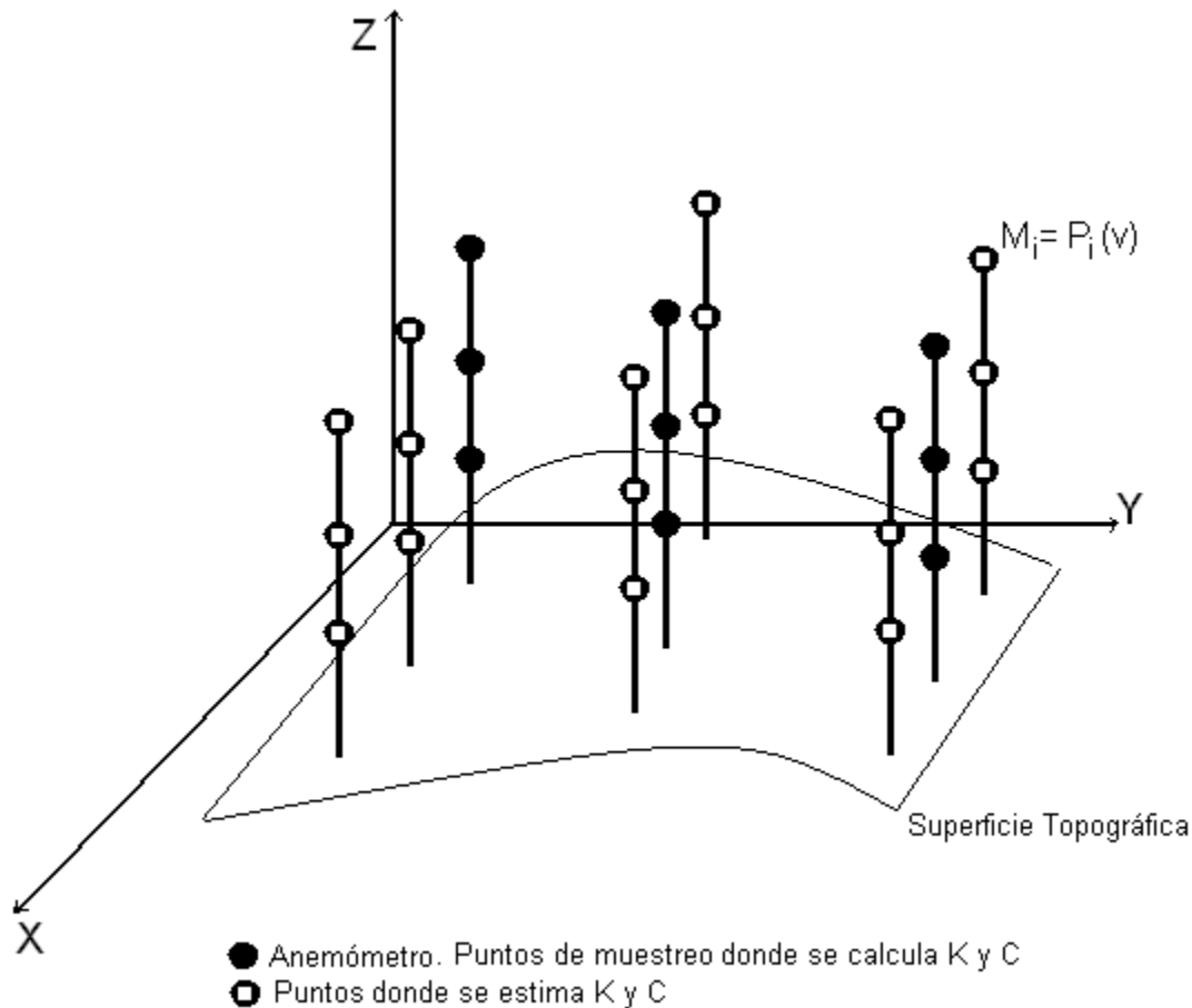
Figura 1: Modelo del potencial eolo-energético con m=54 puntos 3D cuyo muestra consta de n=9 puntos.
